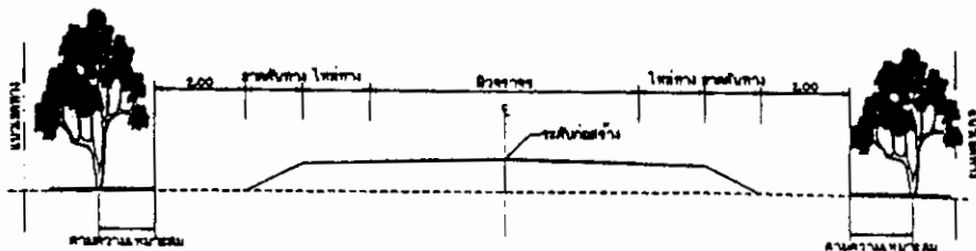
รูปตัดแสดงการปลูกต้นไม้ 2 ช่องทาง
