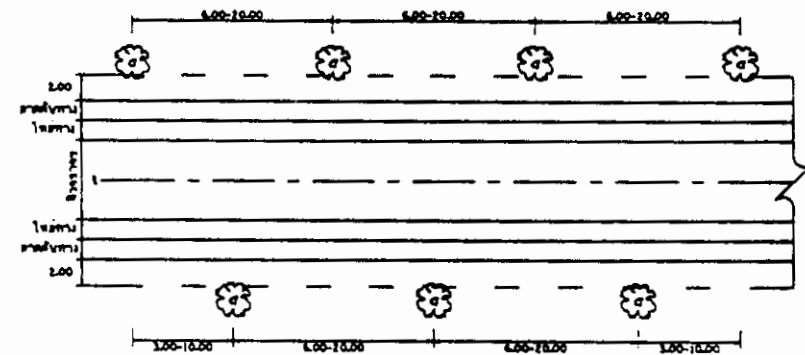
แผนแสดงระยะการปลูกต้นไม้ 2 ช่องทาง
