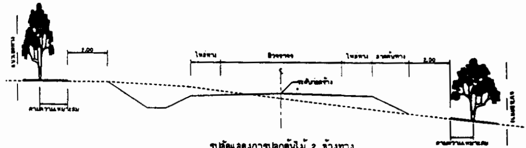
รูปตัดแสดงการปลูกต้นไม้ 2 ช่องทาง กรณีที่เป็นสันดินและดินถม
